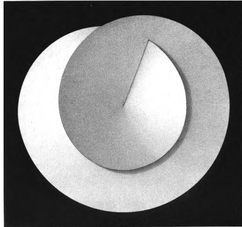
Die Riemann'sche Windungsfläche erster Ordnung
